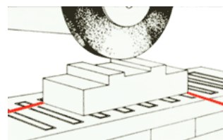
Indretning af emne
