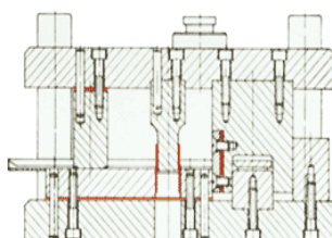
For måling af frigang i skærende værktøjer
